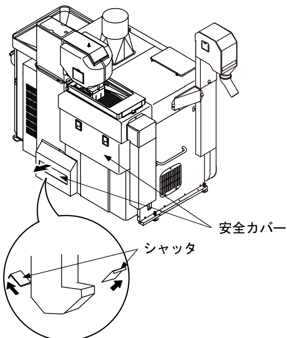
混合昇降機掃除口 (左右2カ所)
