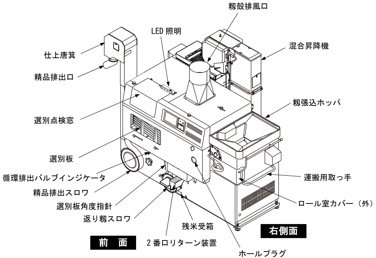
図 3 機械全体図 (1)
