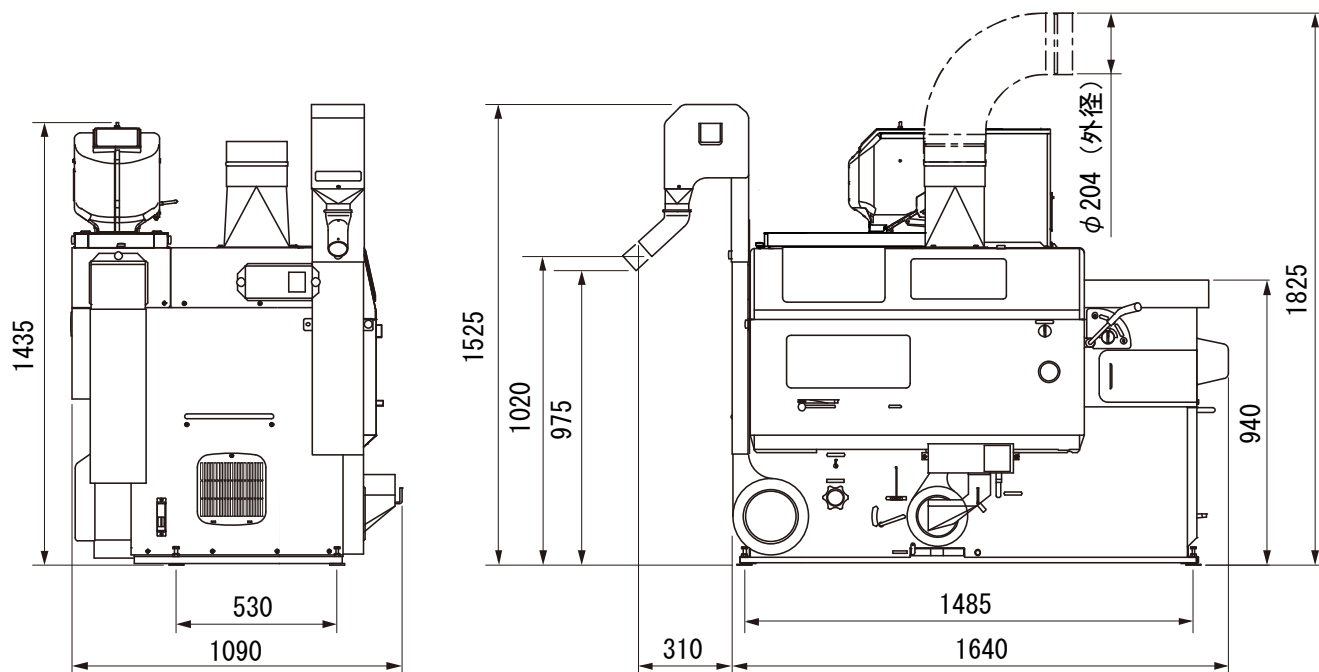
図 8 機体寸法
