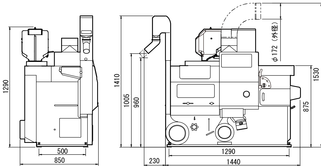
図 9 機体寸法
