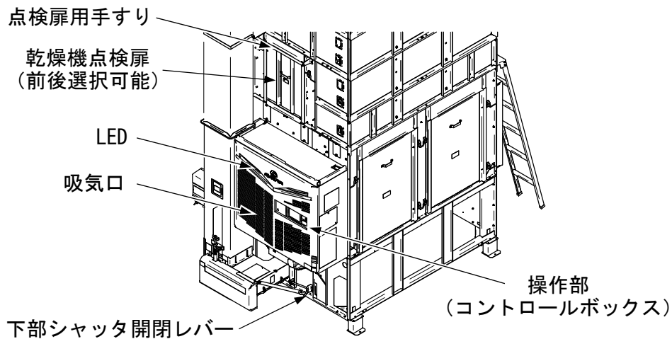
図 3 機械全体図 (1)
