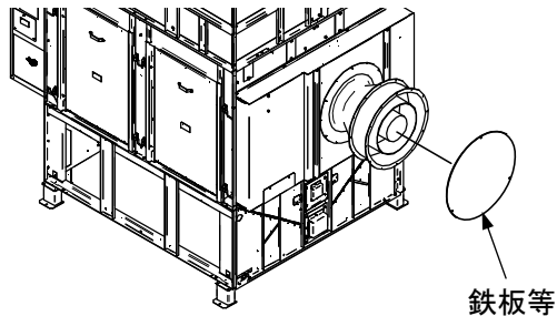
斜流式 2.0kW 送風機
