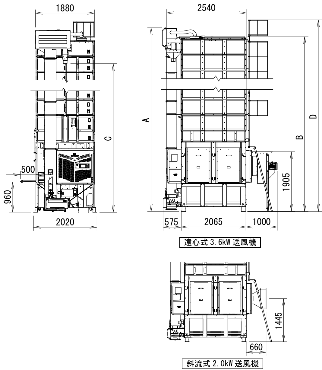
図 5 機体寸法
