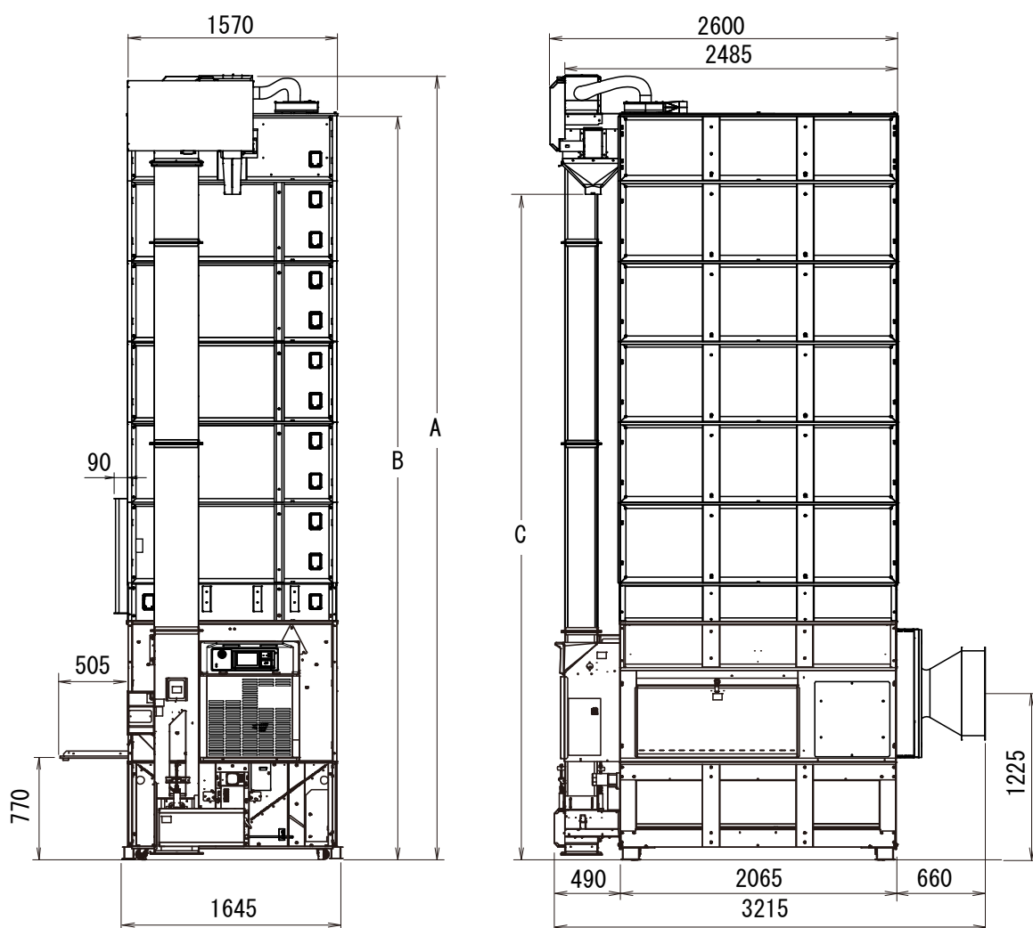
図 5 機体寸法
