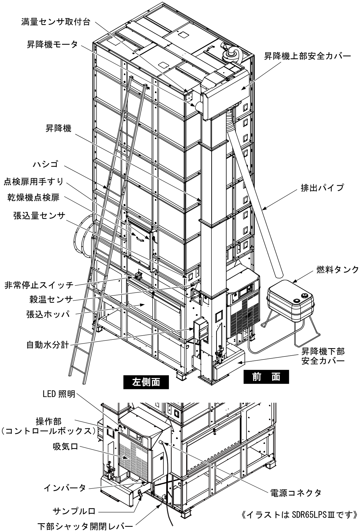
図 3 機械全体図 (1)
