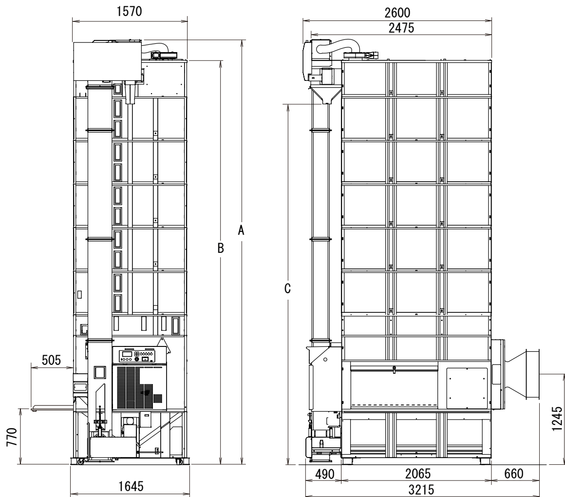
図 5 機体寸法
