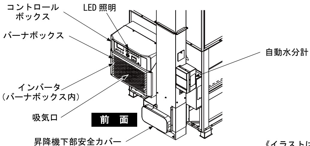
図 3 機械全体図 (1)
