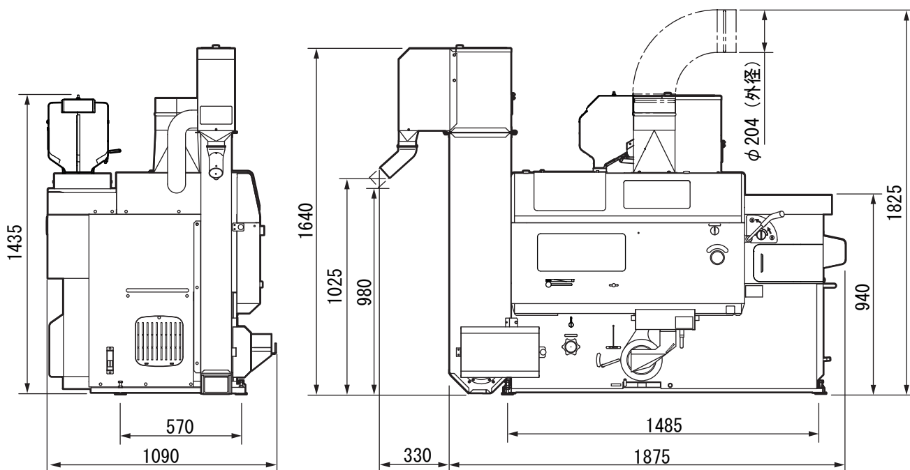
図 9 機体寸法
