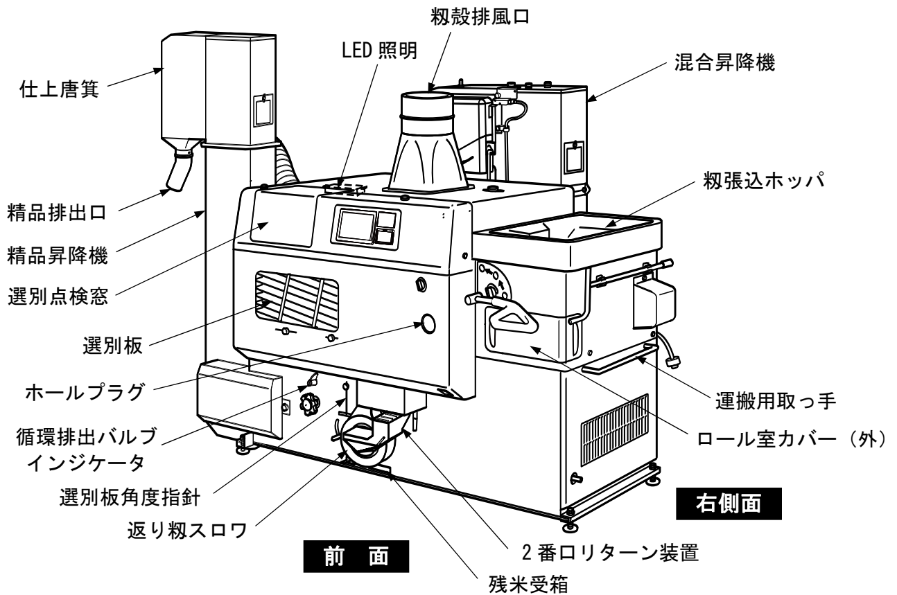
図 3 機械全体図(1)
