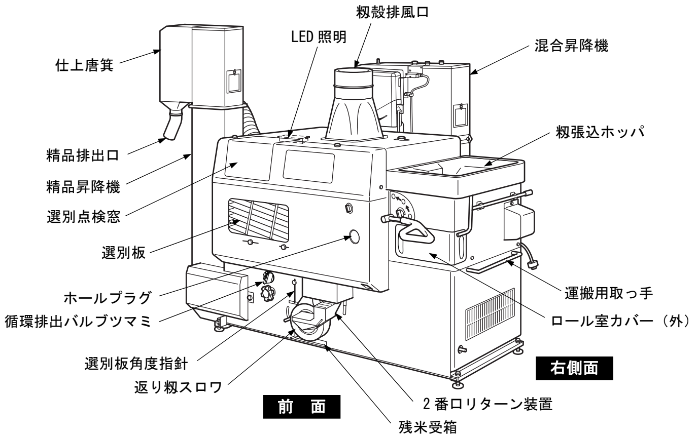
図 3 機械全体図 (1)
