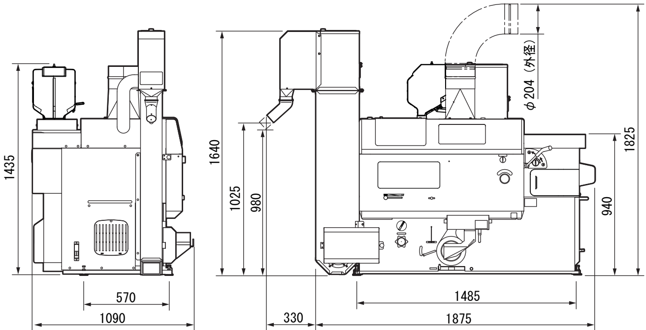
図 9 機体寸法
