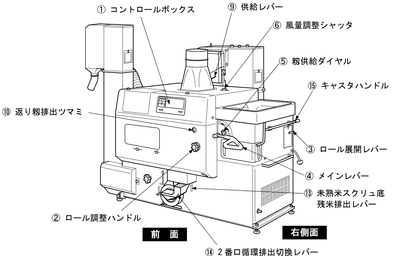
図 5 機械操作箇所 (1)
