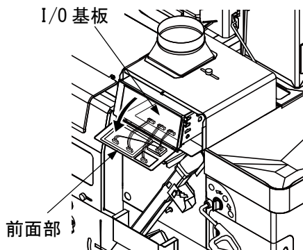
※I/O 基板を上から見た図
