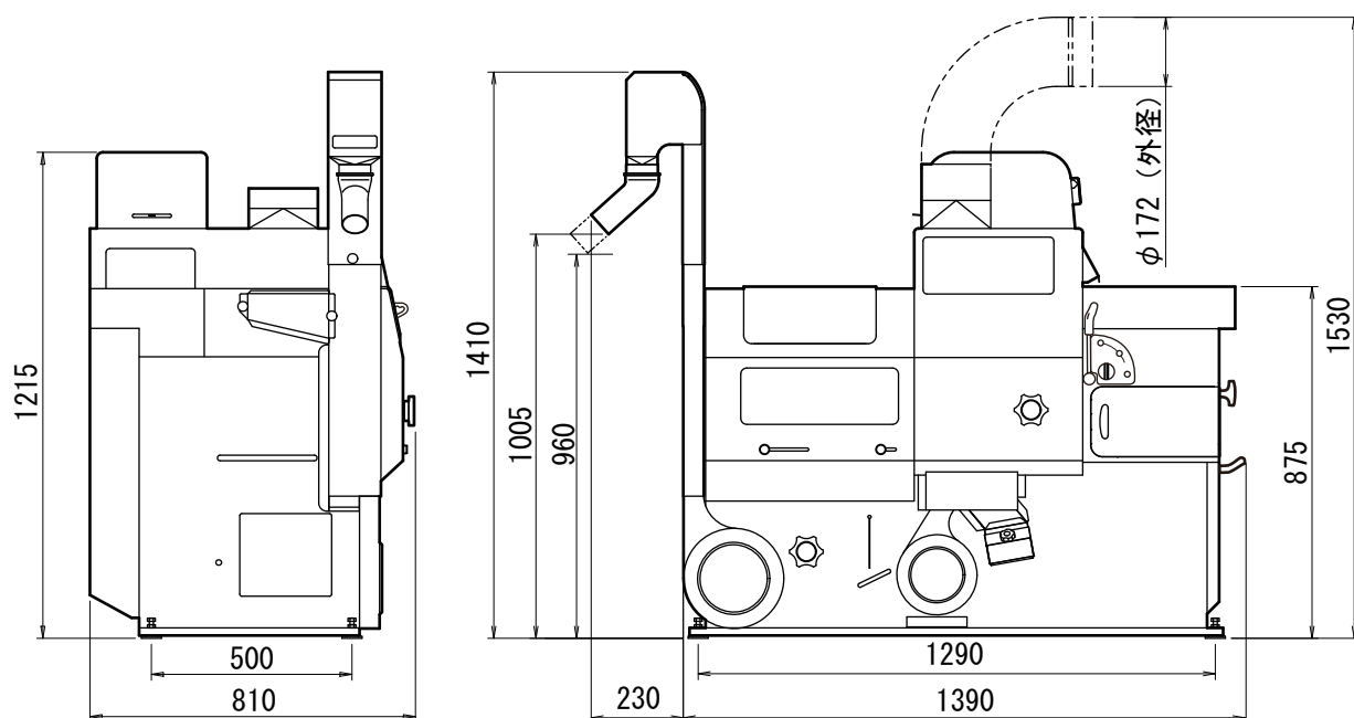
図 7 機体寸法
