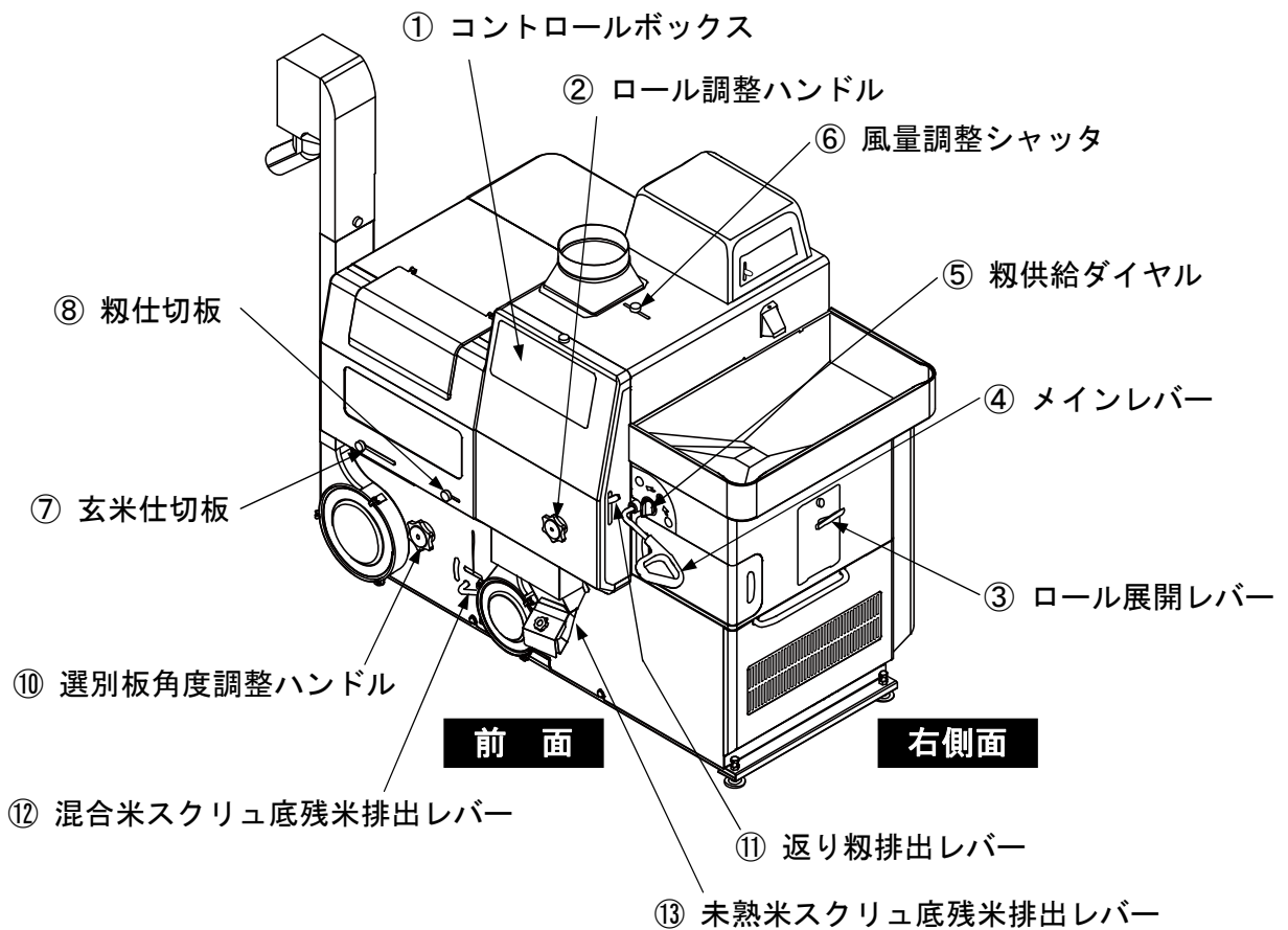
図 5 機械操作箇所 (1)
