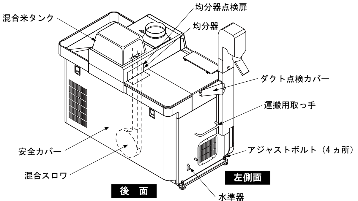
図 4 機械全体図 (2)
