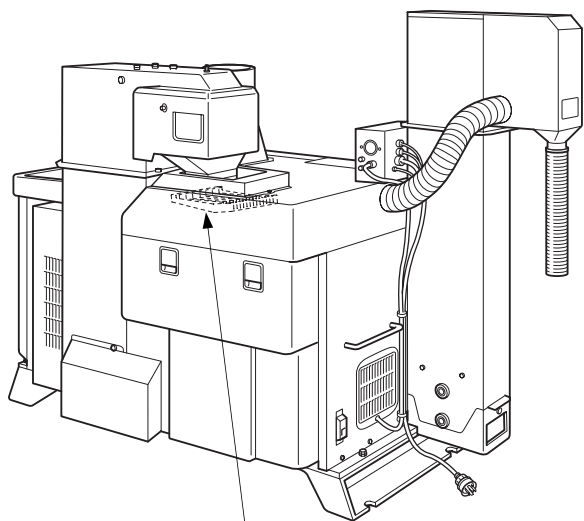
粗選スクリーン
