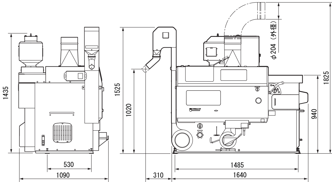
図 9 機体寸法
