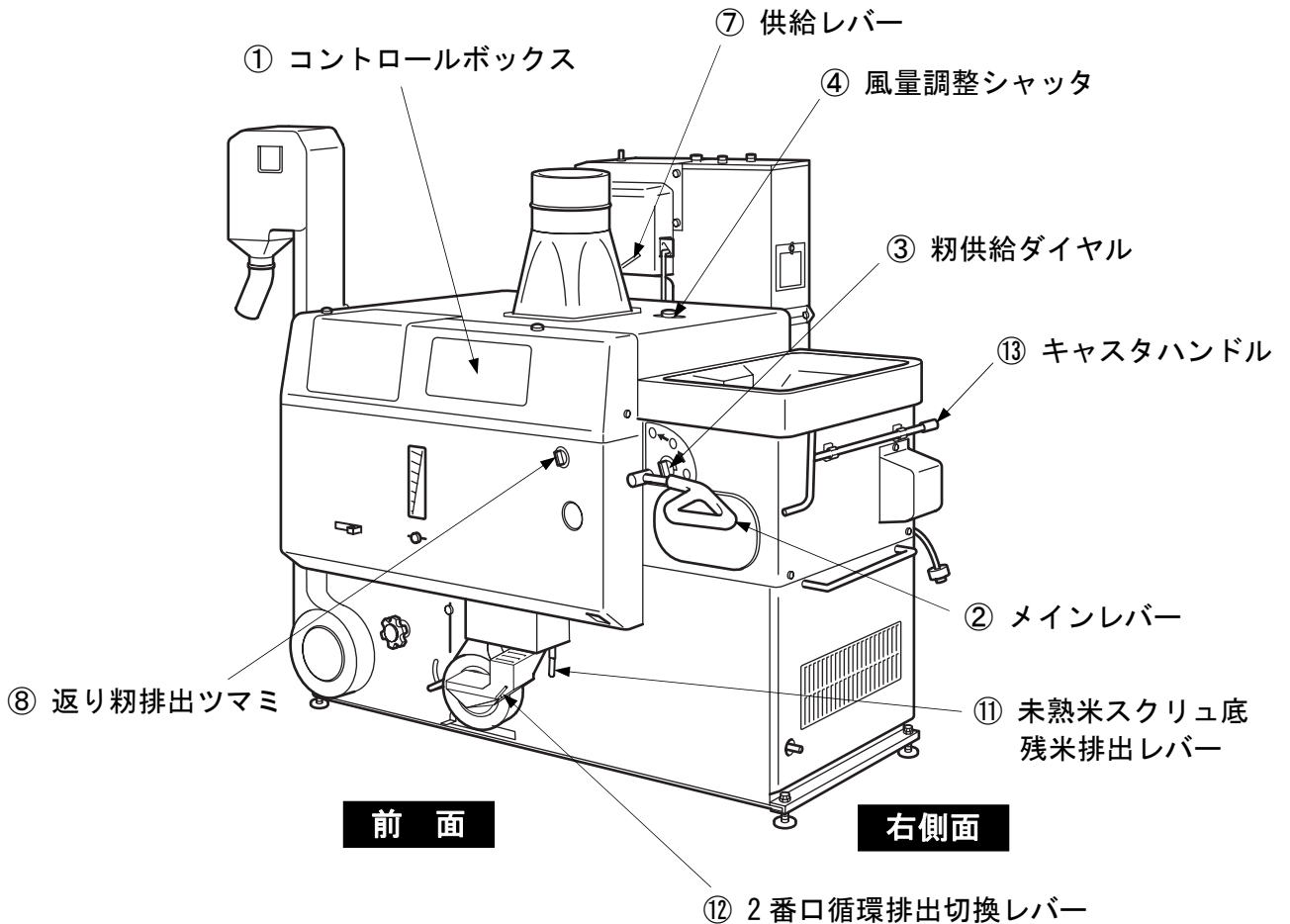
図 6 機械操作箇所 (1)
