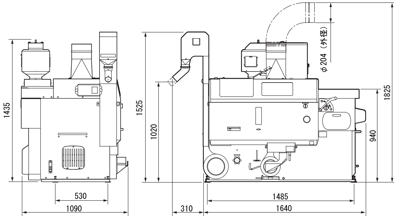
図 8 機体寸法
