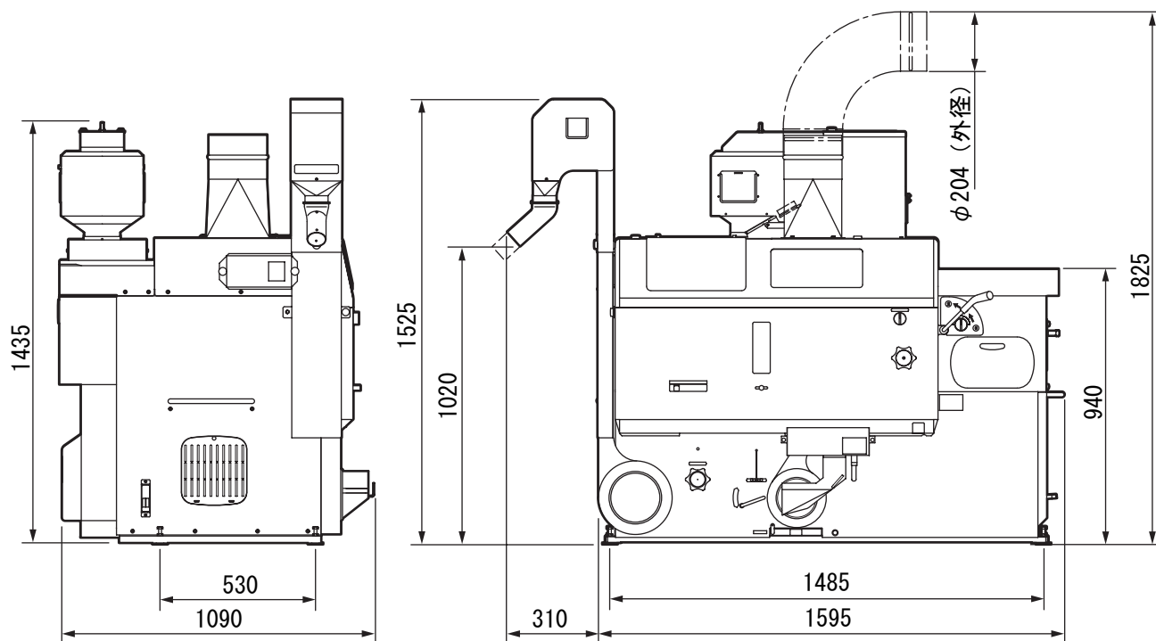
図 7 機体寸法
