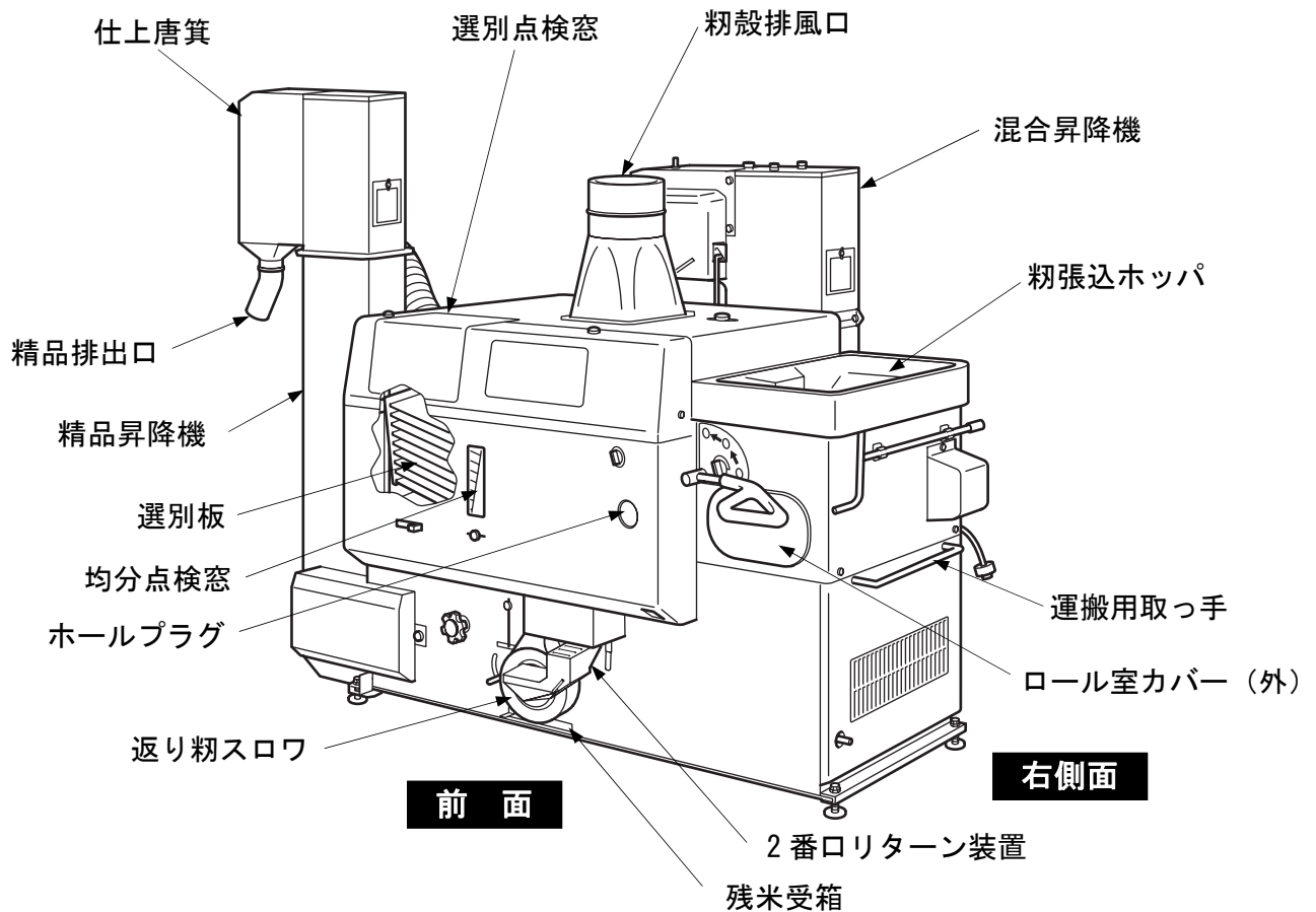
図 3 機械全体図 (1)
