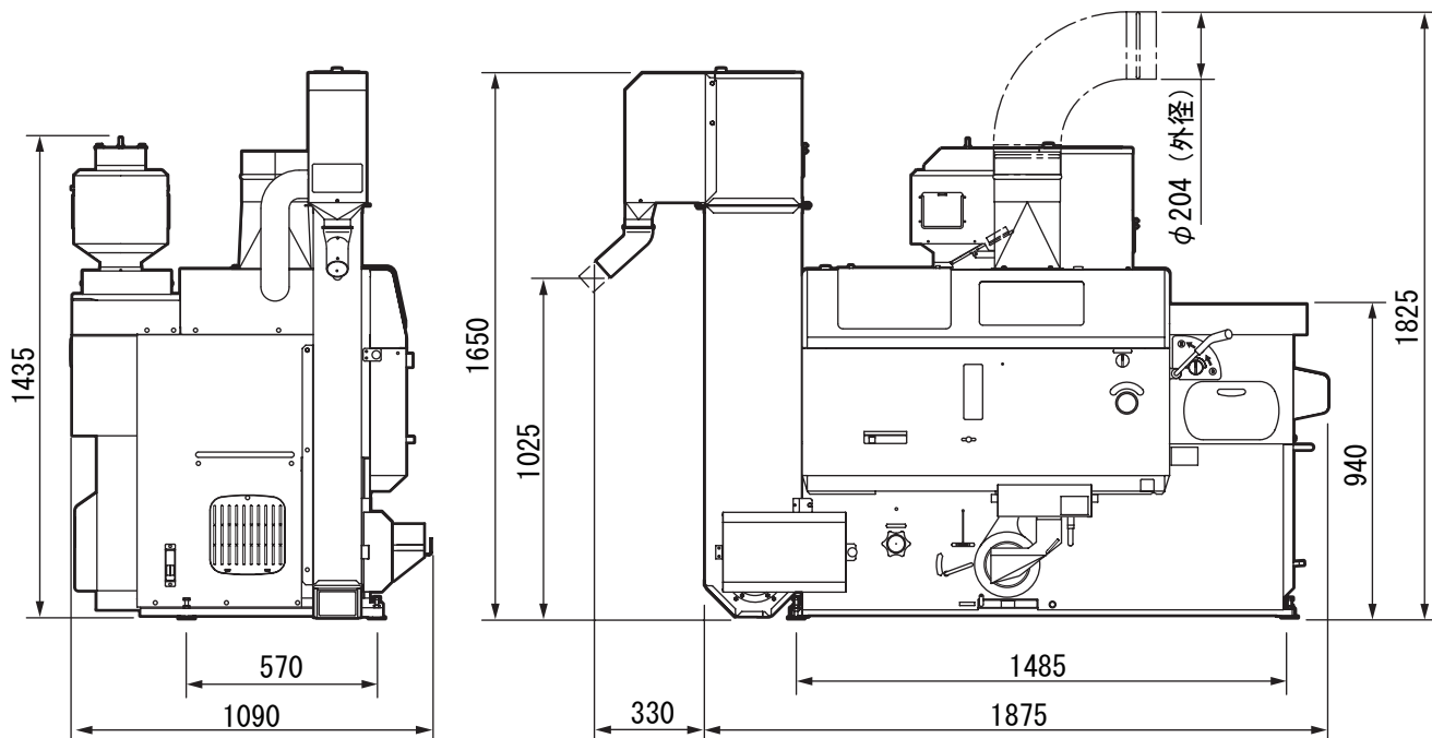
図 8 機体寸法
