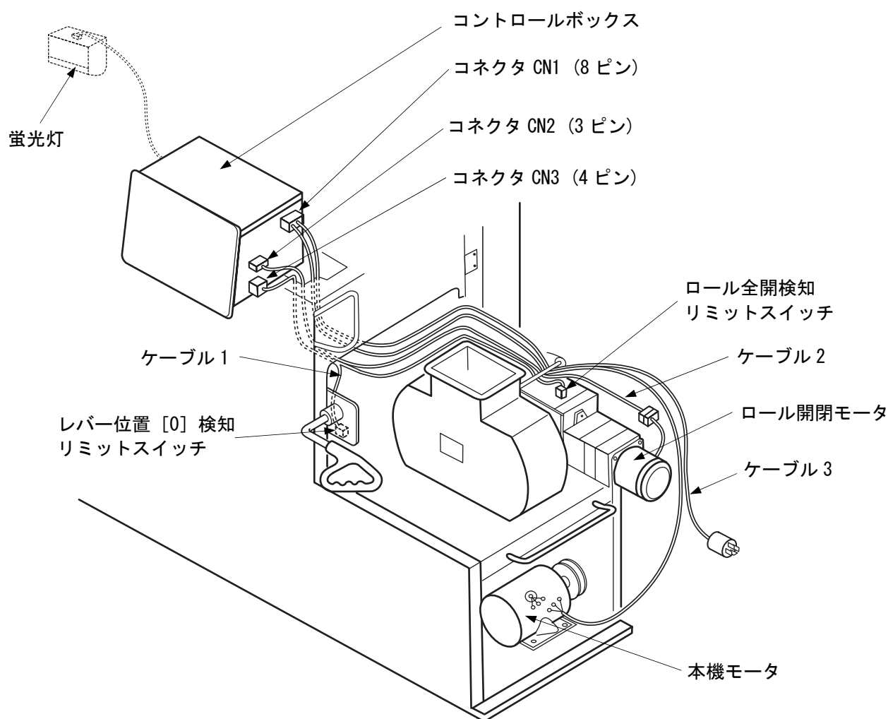
図 5 電装部品の構成
