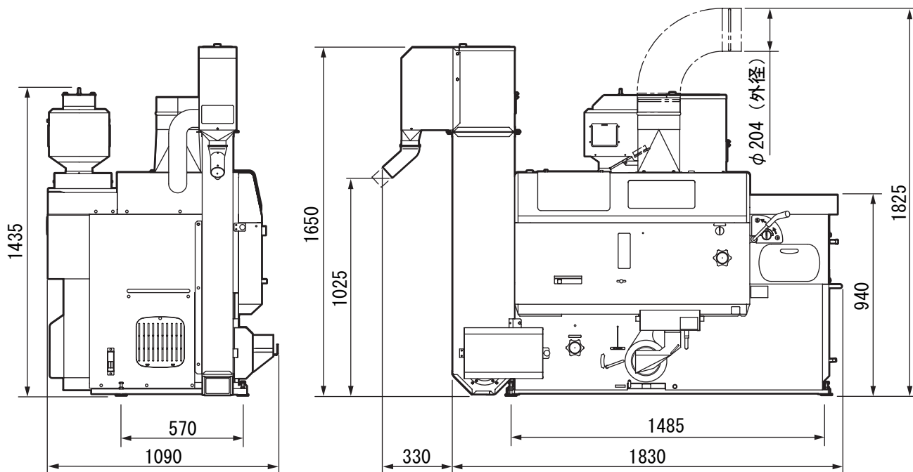
図 7 機体寸法
