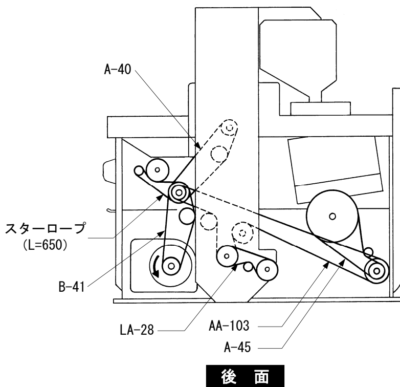
図 9 ベルトの掛け方とサイズ
