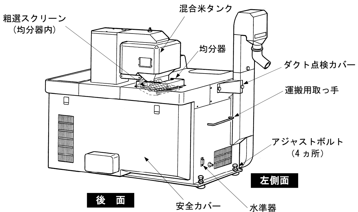
図 4 機械全体図 (2)
