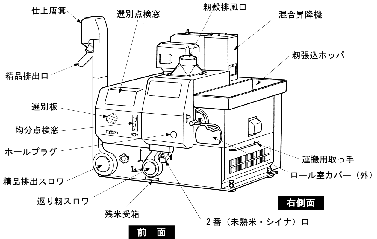
図 3 機械全体図 (1)
