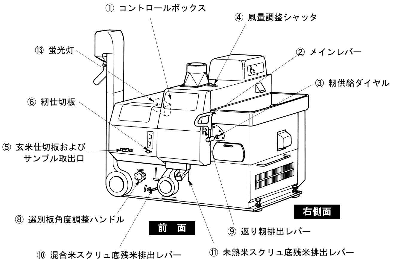
図 6 機械操作箇所 (1)
