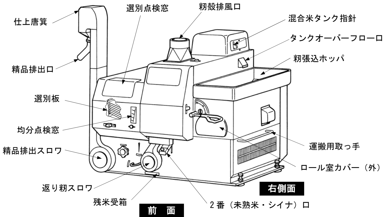
図 3 機械全体図 (1)
