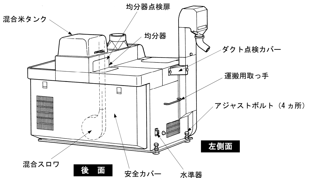
図 4 機械全体図 (2)
