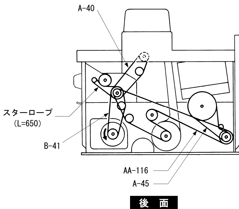
図 9 ベルトの掛け方とサイズ
