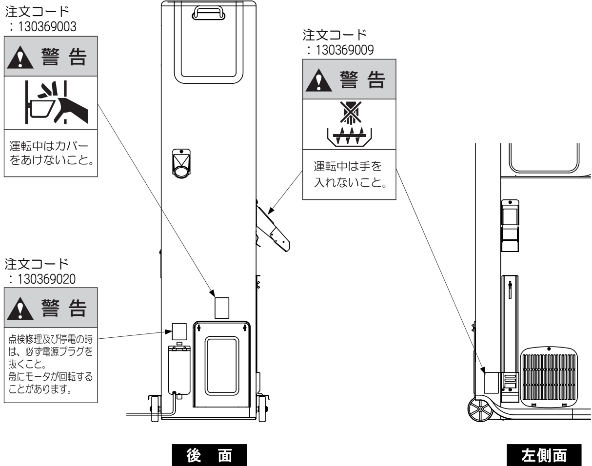
図 2 標示ラベル貼付位置 (2)
