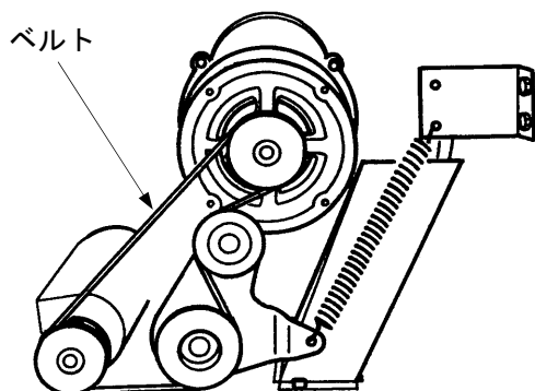
図は底から見た状態です
