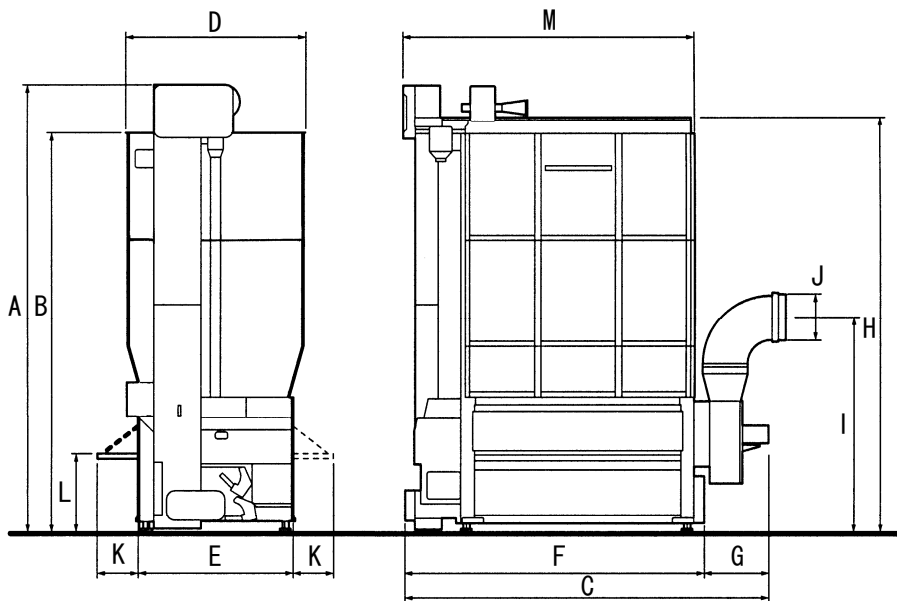
図 11 GDR15・18・21・24・27SZG 機体寸法
