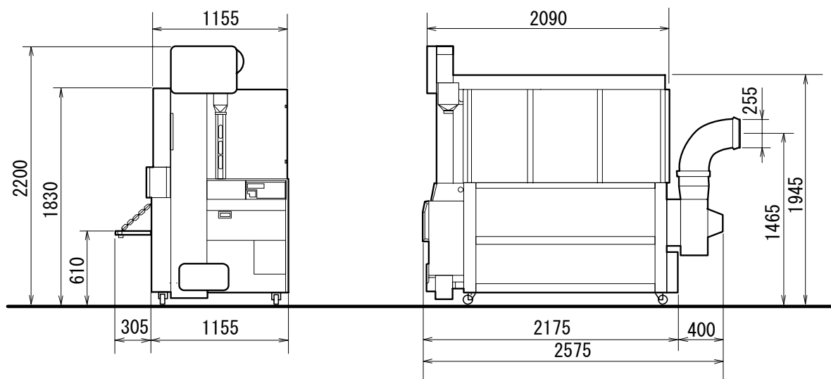
图 12 GDR9VZG 機体寸法
