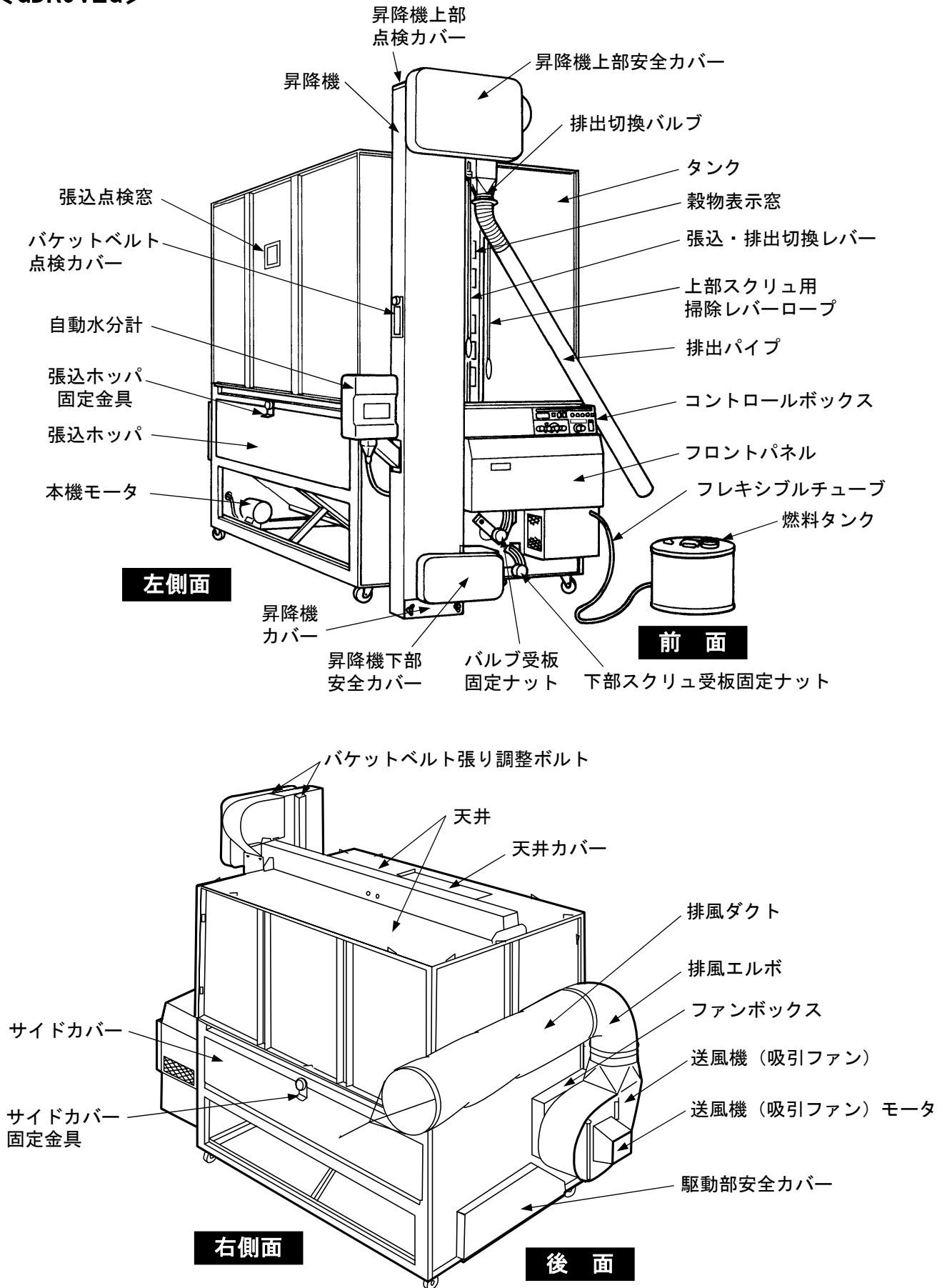
図 5 機械全体図 (3)
