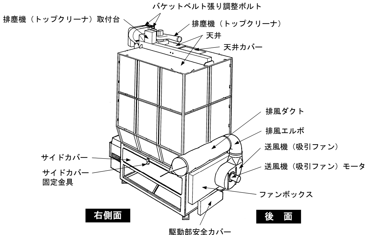
図 4 機械全体図 (2)
