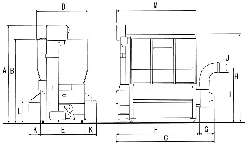
図 10 GDR11・13・14SZG 機体寸法
